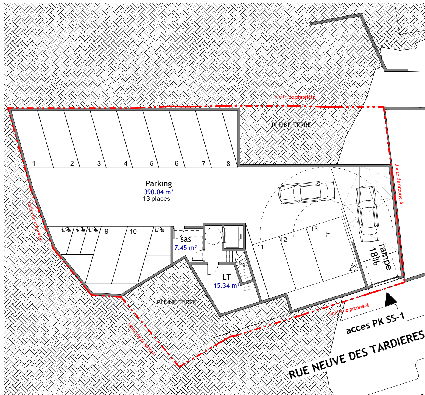
Niveau S1 Ech : 1 : 200
